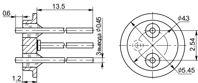
Основание КЮЯЛ.432264.115
