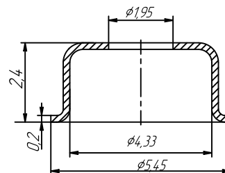
Колпак КЮЯЛ.725213.035
